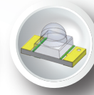
SMD 3216-18 3.20*1.60*1.86mm
