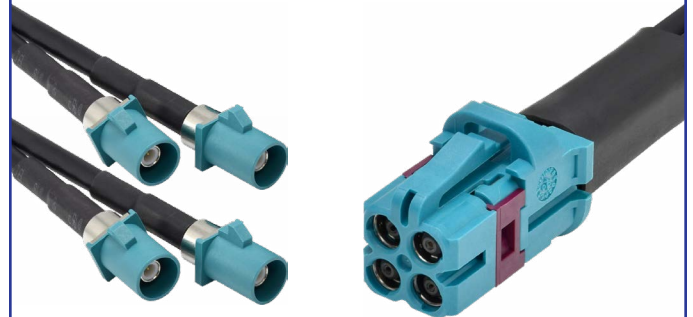
Mini FAKRA Straight Jack to 4 Standard FAKRA Straight Plugs Cable
