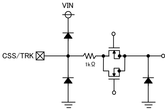
< CSS/TRK Pin >
