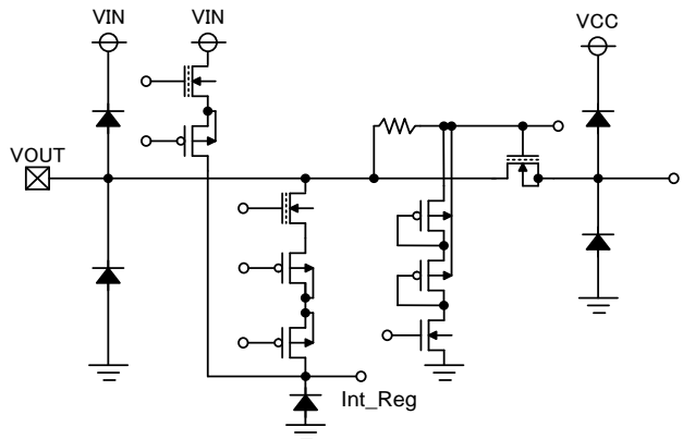
< VOUT Pin >
