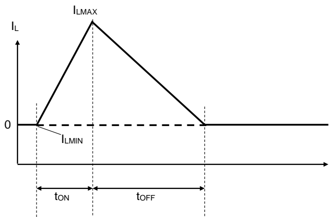
VFM Mode
