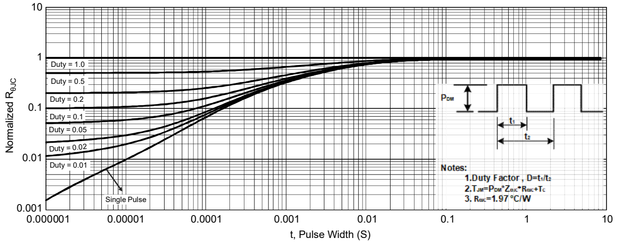
FIG. 7-Transient Thermal Impedance
