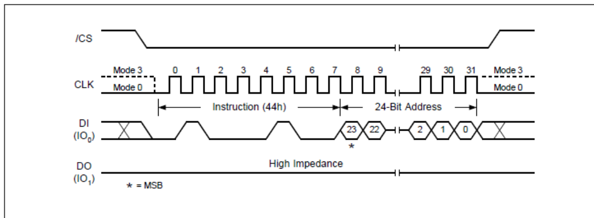
Erase OTP array
