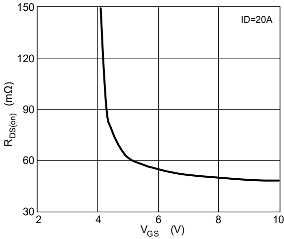
FIG. 1- R_{DS(on)} vs. V_{GS}
