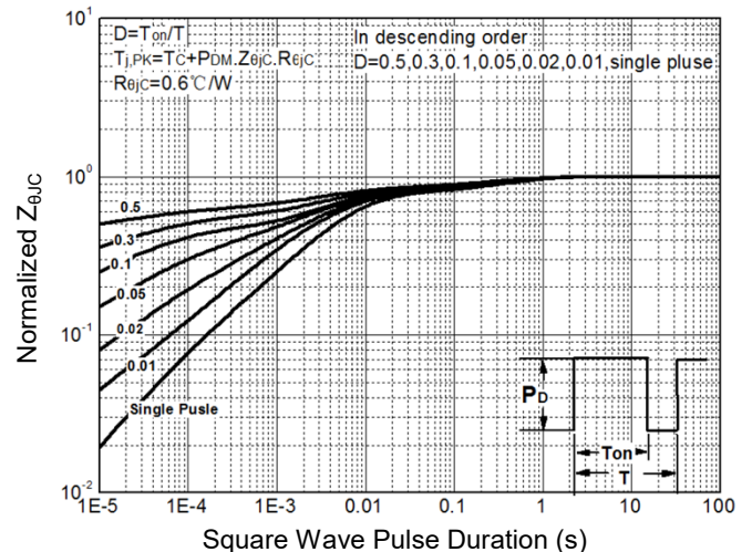
FIG. 6 - Thermal Transient Impedance
